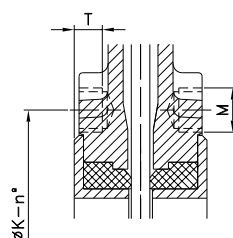
DN 450-600
